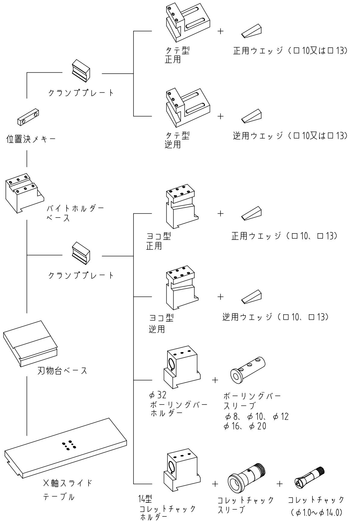
図7 ツーリングシステム
